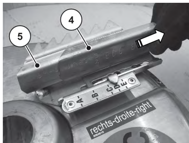
Fig. 84: Förlängnings- och huvudvinge
