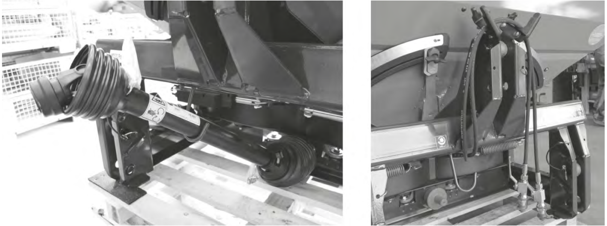
Fig. 64: Kraftöverföringsaxelns förvaring, kablarnas förvaring och hydraulslangar
