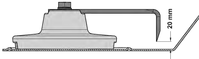
Fig. 77: Omrörarfingrets slitageområde
