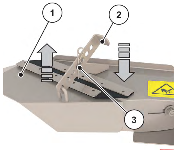
Fig. 63: Justering på radspridningsutrustningen
