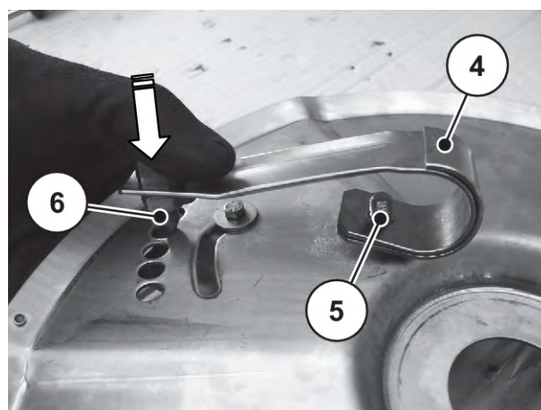
Fig. 95: Plan fjäder på spridartallriken
