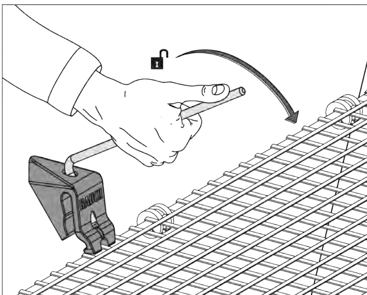
Fig. 68: Öppna skyddsgallerlåsen
