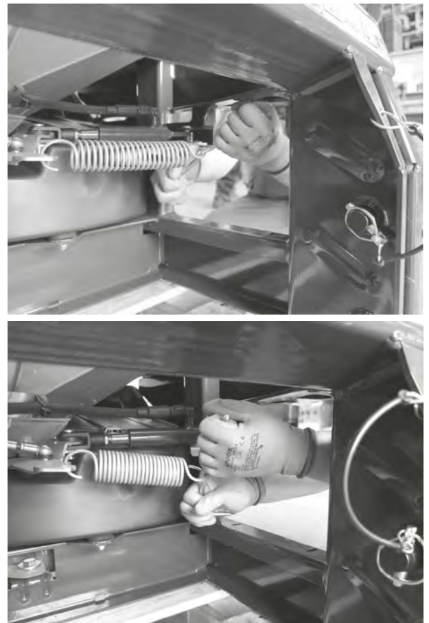
Fig. 71: Haka ur fjädern
