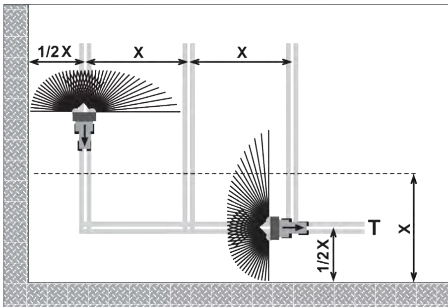
Fig. 59: Gränsspridning
