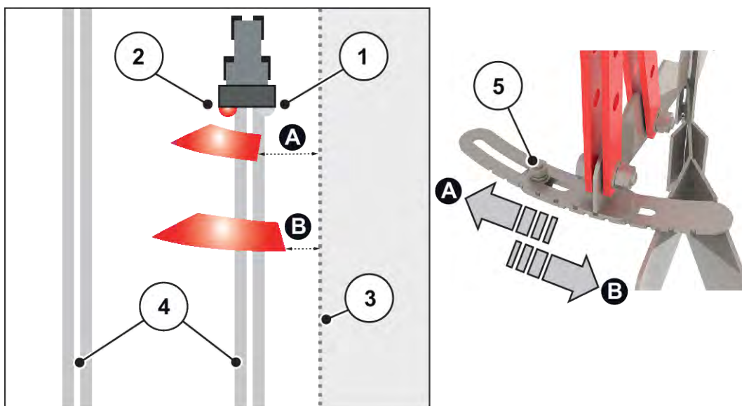
Jn. 56: Piiripuisteseadise seadistus
