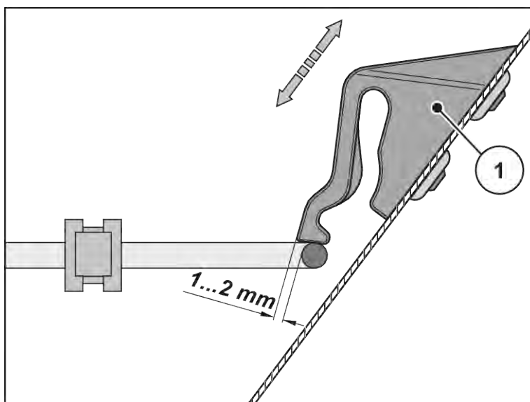
Jn. 69: Kaitsevõre lukustuse talitluskontrolli kontrollimõõt
