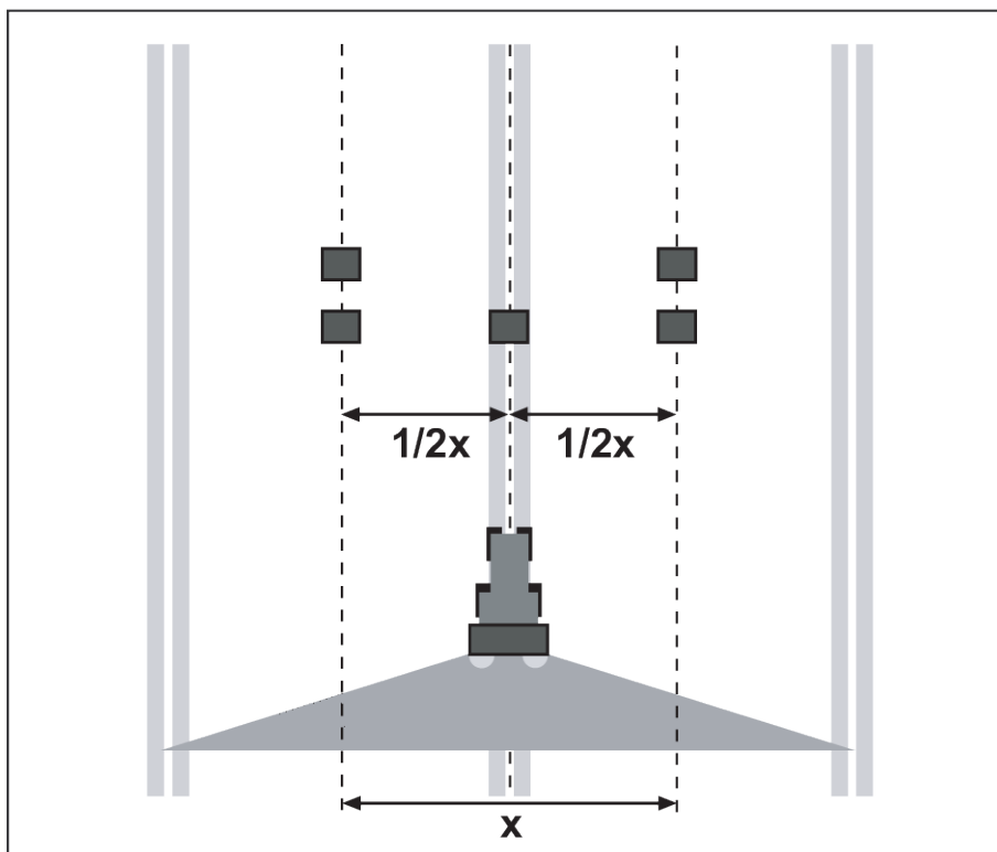
Jn. 53: Ülesseadmine ühe ülesõidu jaoks
