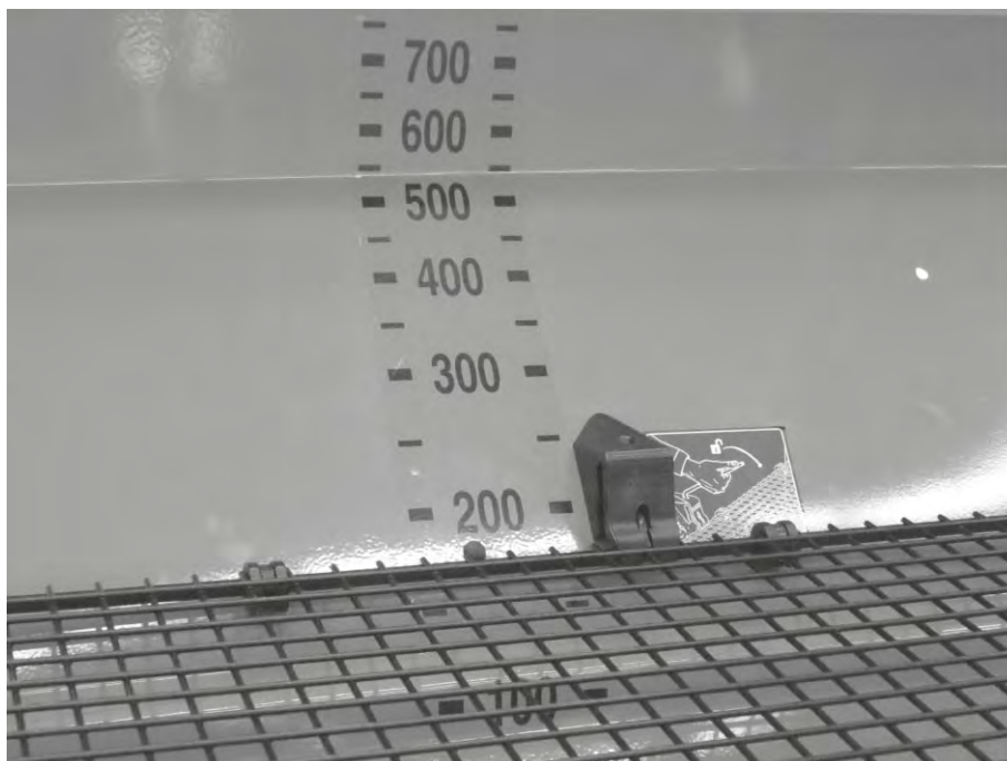
Рис. 30: Шкала уровня заполнения (данные в литрах)
