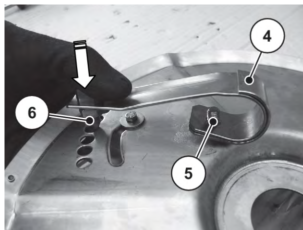
Рис. 93: Плоская пружина на разбрасывающем диске
