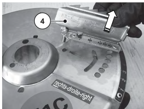
Рис. 89: Снятие лопатки для разбрасывания
