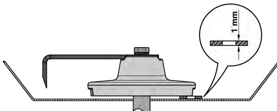
Рис. 78: Настройка мешалки
