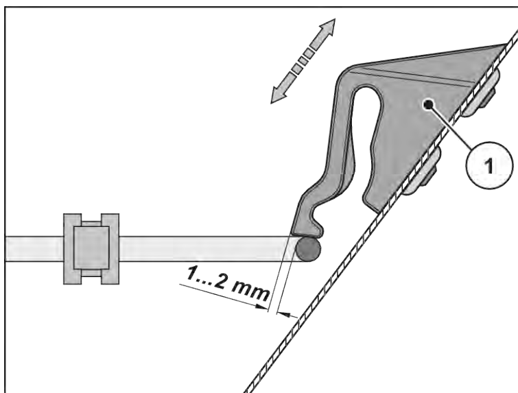
Рис. 67: Контрольный размер для проверки функционирования блокировочного устройства защитной сетки
