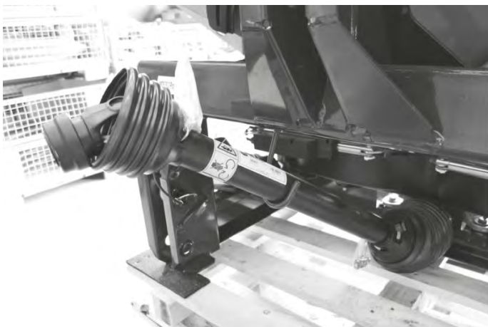
Рис. 62: Место размещения карданного вала, кабелей и гидравлических шлангов
