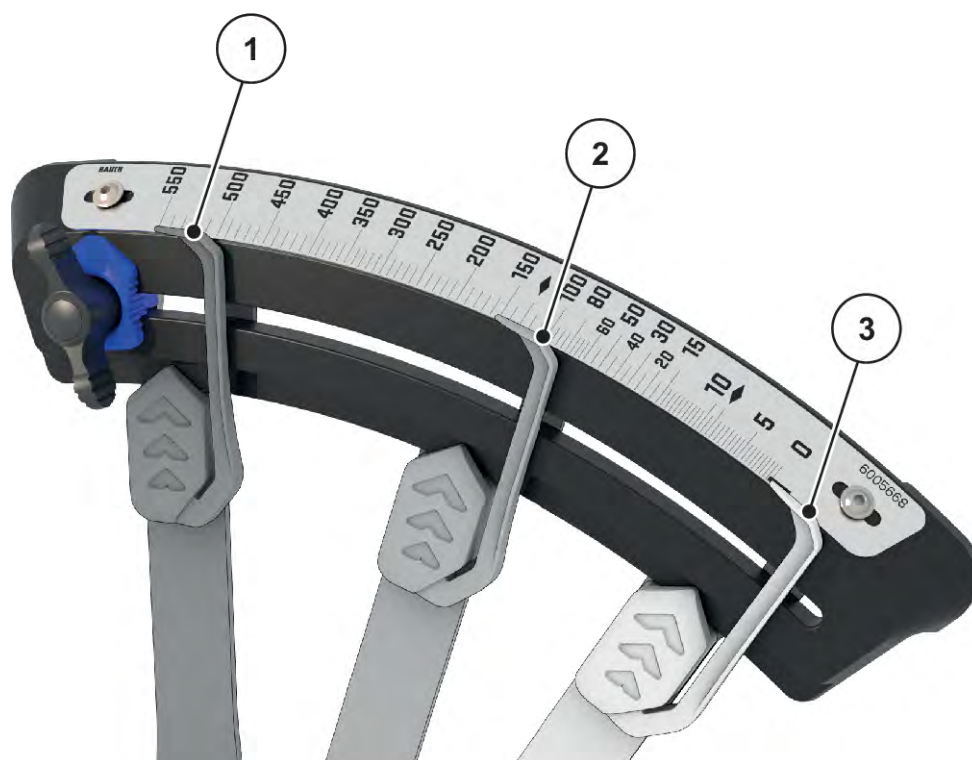
Рис. 29: Положения заслонки дозатора
