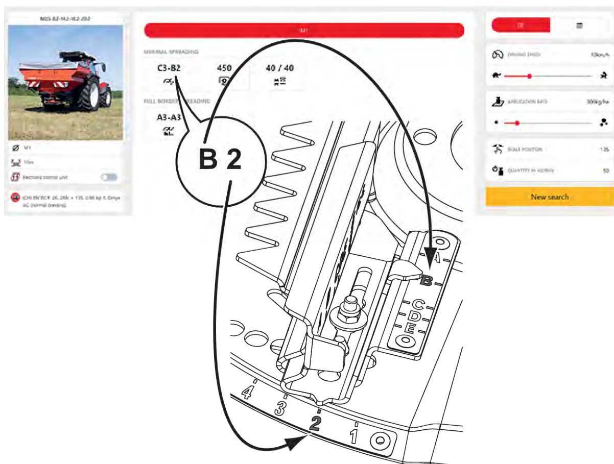
Рис. 41: Регулировка лопатки для разбрасывания; положение B2; от A до E: Регулировка длины от 1 до 6: Регулировка угла
