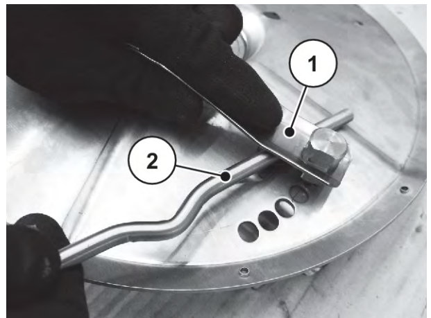
Рис. 87: Снятие плоской пружины
