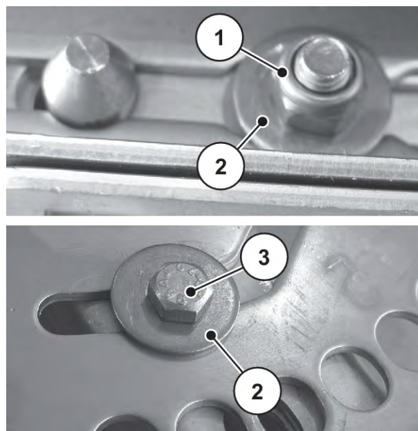
Рис. 92: Точки крепления лопаток для разбрасывания
