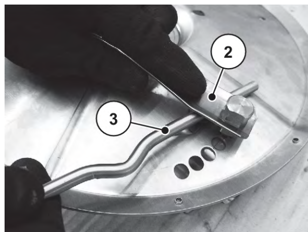
Рис. 81: Разблокирование плоской пружины
