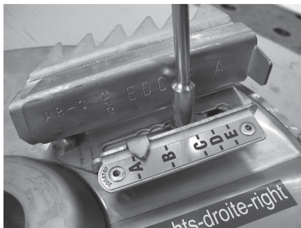
Рис. 91: Лопатки на разбрасывающем диске
