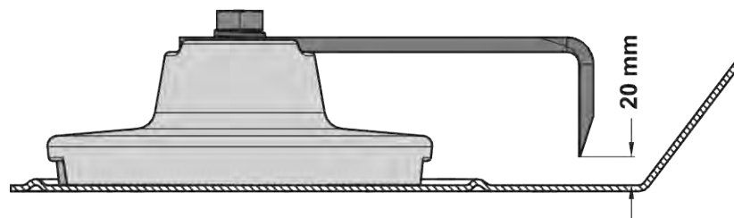
Рис. 75: Область износа лопасти мешалки
