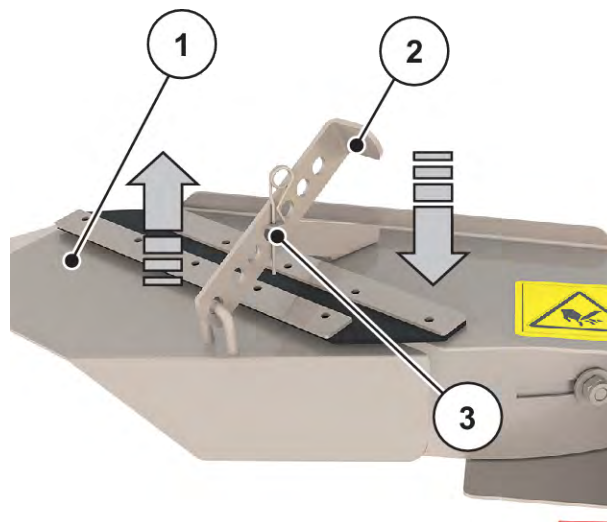
Рис. 61: Регулировка на приспособлении для внесения по рядам
