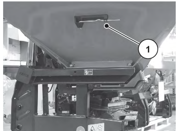
Рис. 34: Положение регулировочного рычага
