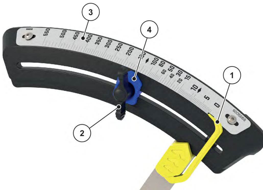
Рис. 39: Шкала для настройки количества вносимого удобрения (справа по направлению движения, варианты K/D/C)
