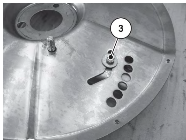
Рис. 88: Винт на нижней стороне разбрасывающего диска
