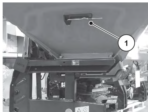
Рис. 8: Расположение регулировочного рычага
