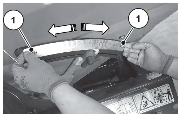
Рис. 74: Перемещение шкалы
