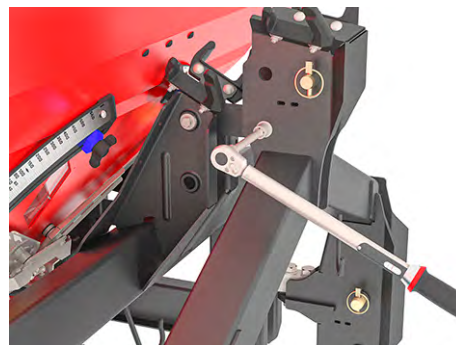
Рис. 64: Крепление растянутого стержня на раме для взвешивания
