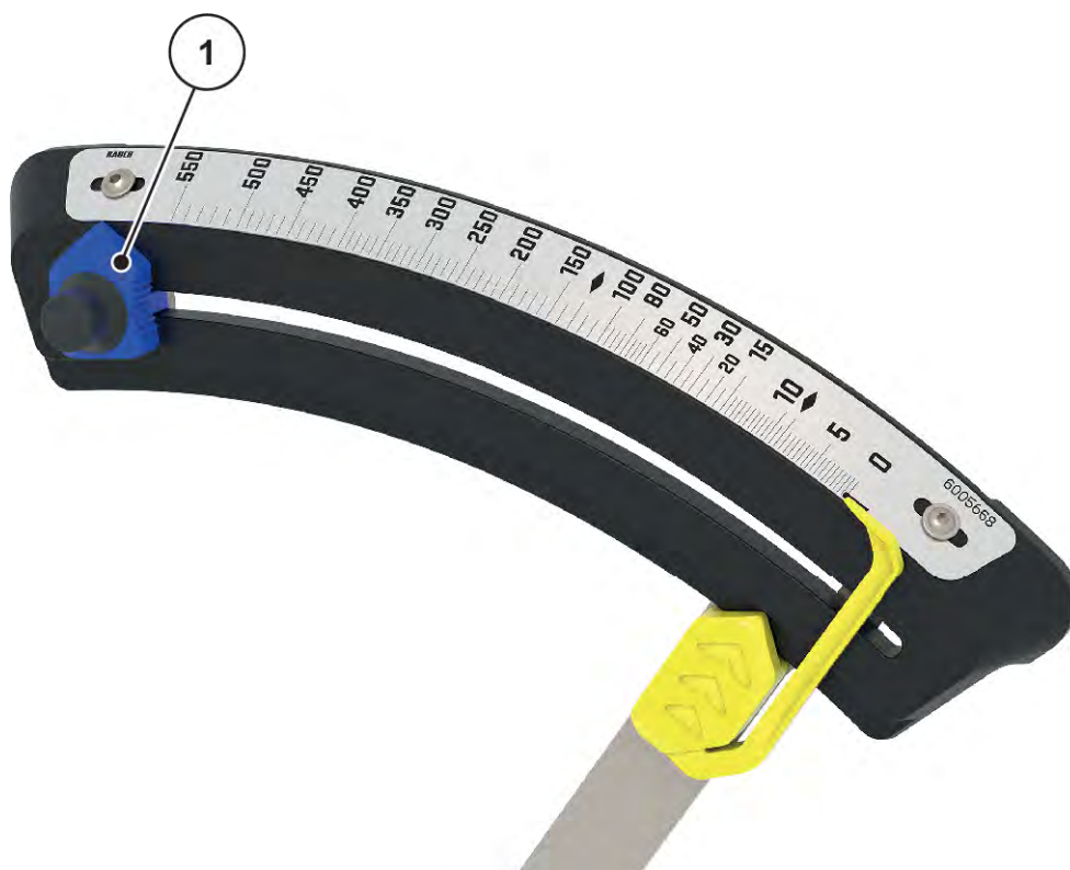
Рис. 40: Шкала для настройки количества вносимого удобрения (справа по направлению движения, вариант Q)
