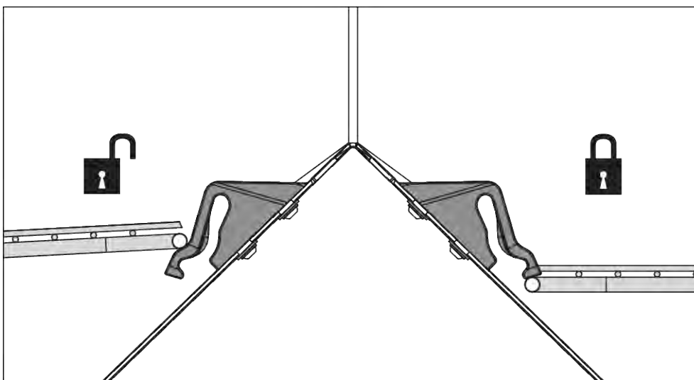
Рис. 65: Блокировочное устройство защитной сетки открыто/закрыто
