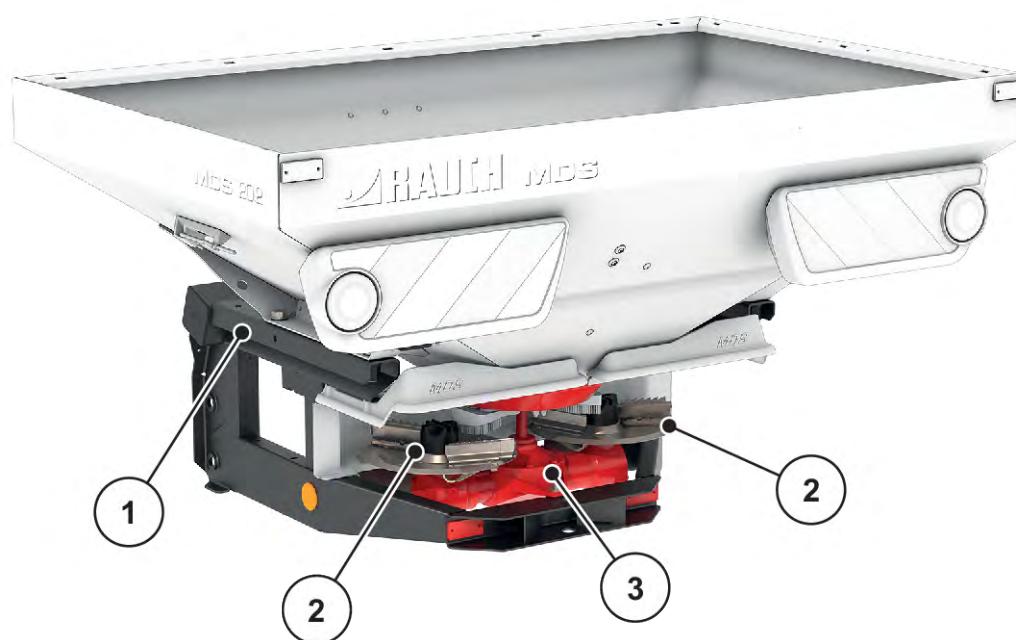
Рис. 7: Обзор конструктивных узлов: Задняя сторона
