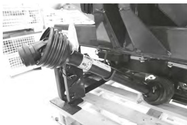
Рис. 16: Крепление карданного вала
