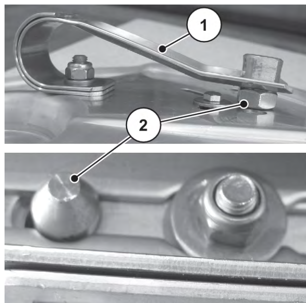
Рис. 77: Фиксатор правильно заблокирован
