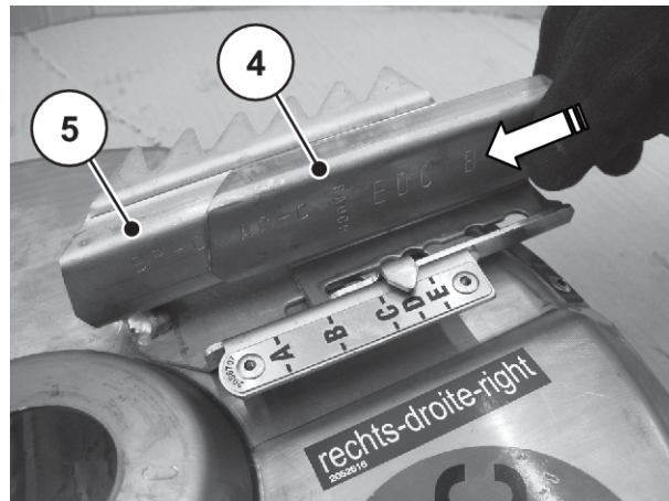
Afb. 85: Nieuwe verlengingsschoep
