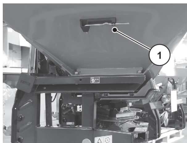
Afb. 36: Positie instelhendel
