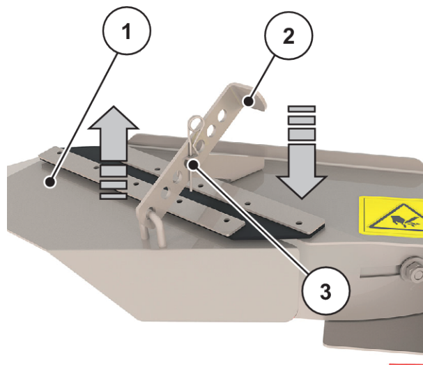
Afb. 63: Verstelling aan de rijenstrooier
