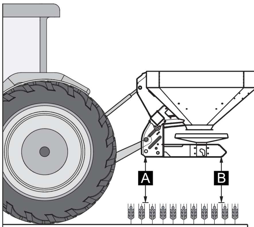
Afb. 24: Aanbouwpositie
