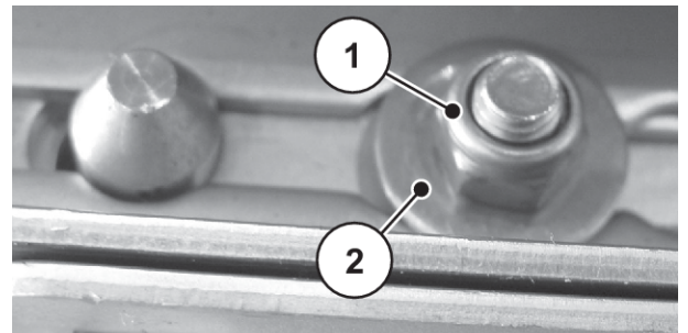
Afb. 93: Strooischoep aan de strooischijf
