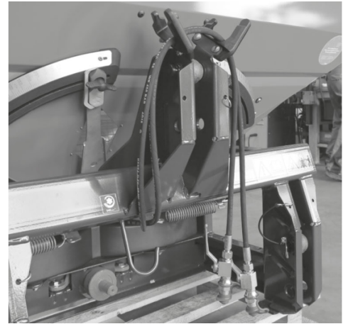
Afb. 64: Neerleggen van de aftakas, neerleggen van de kabels en hydraulische slangen
