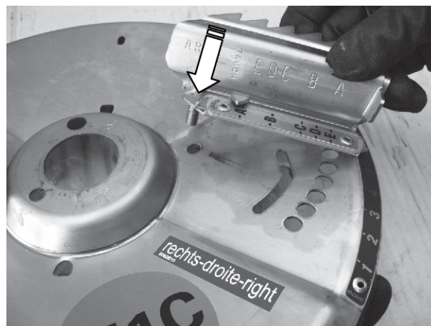
Afb. 92: Hoofdschoepmontage
