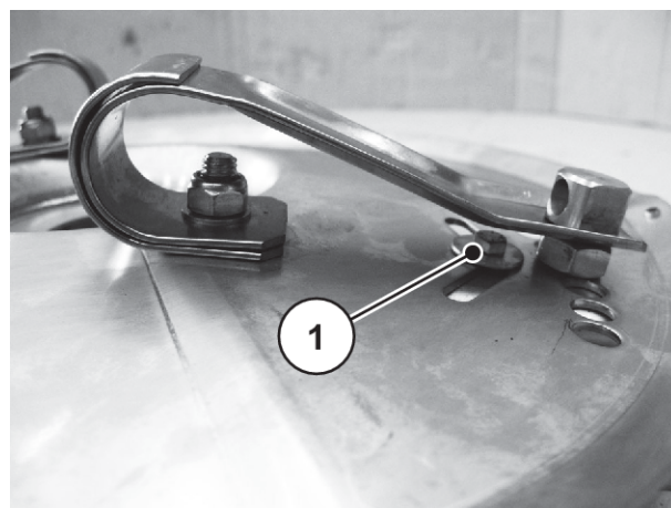
Afb. 82: Platte veer aan de strooischiif
