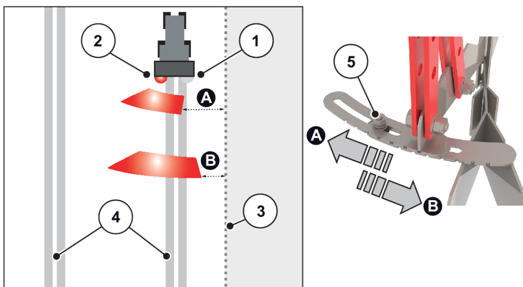
Afb. 56: Instelling van de grensstrooi-inrichting
