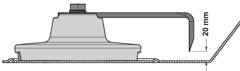
Afb. 77: Slijtagezone van de roerstaaf
