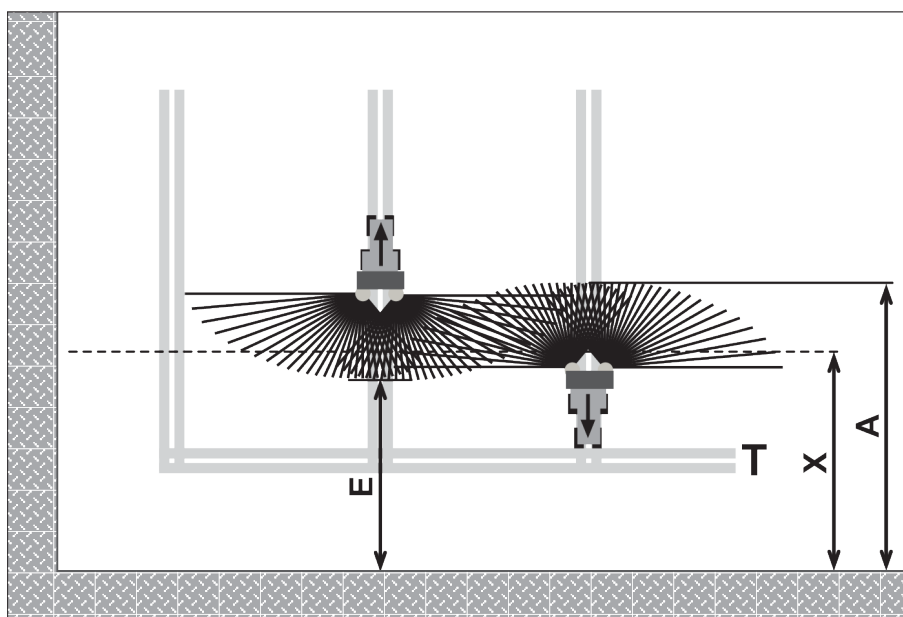
Afb. 60: Normaal strooien
