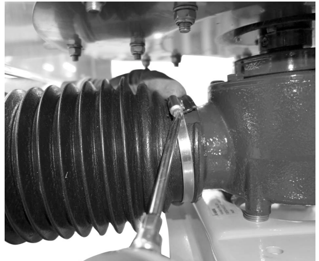
Afb. 16: Aftakasbescherming aanbrengen.
