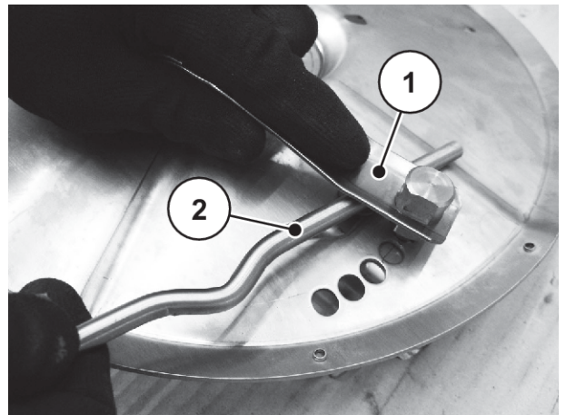
Afb. 89: Verwijderen van de platte veer
