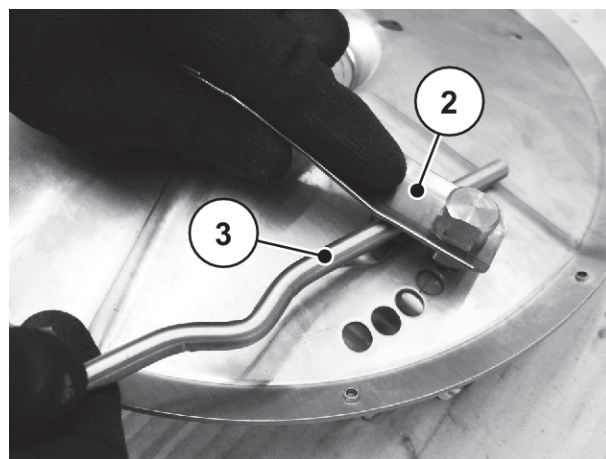
Afb. 83: Platte veer ontgrendelen
