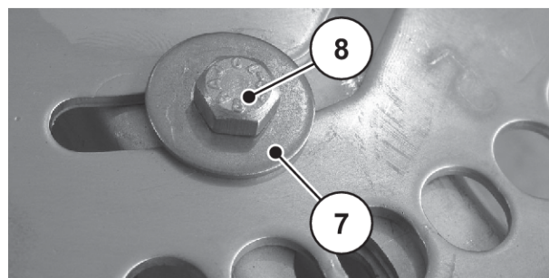
Afb. 86: Bevestigingspunten van de strooischoepen
