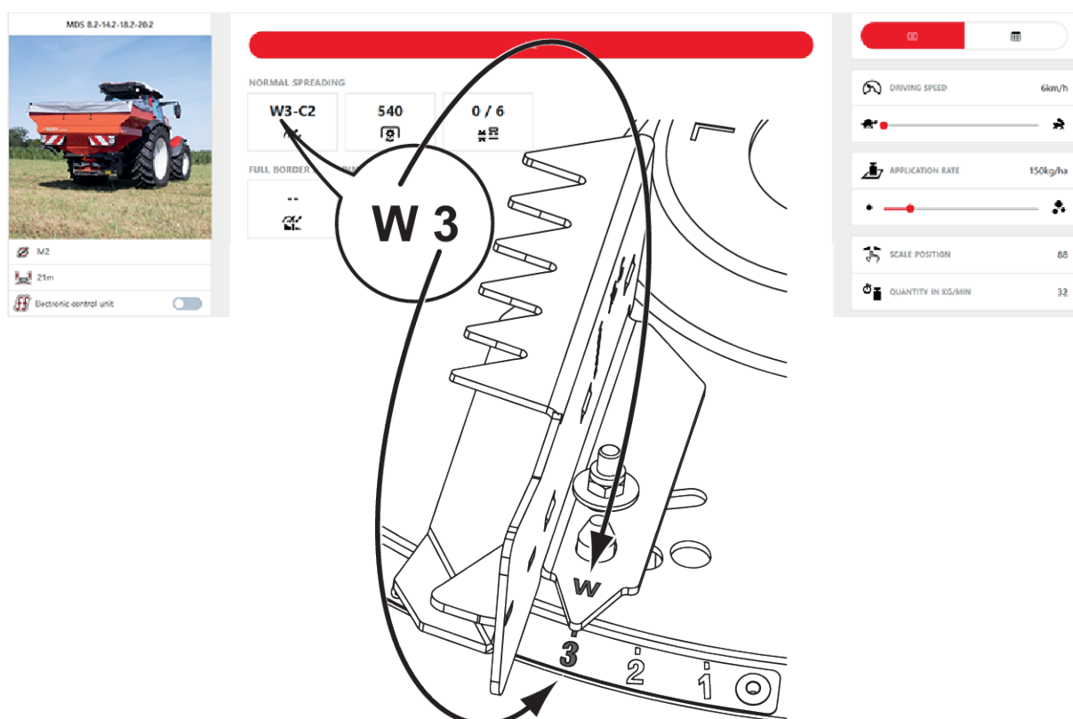
Afb. 44: Strooischoepinstelling strooischoep M2, stand W3; W: vaste lengte-instelling 1 tot 6: hoekinstelling
