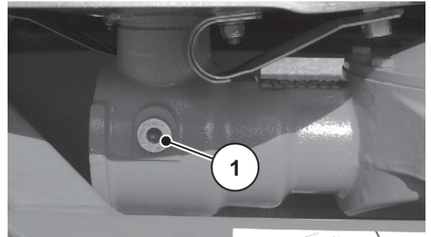
Afb. 97: Vul- en aftappunten voor drijfwerkolie
