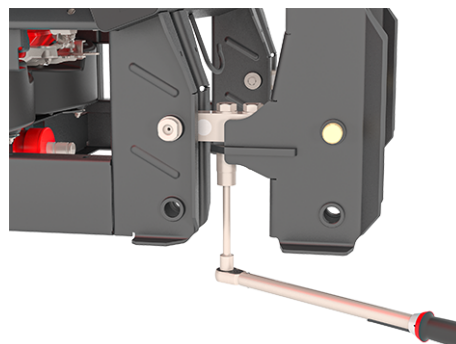
Afb. 65: Bevestiging van de weegcel (in rijrichting rechts)
