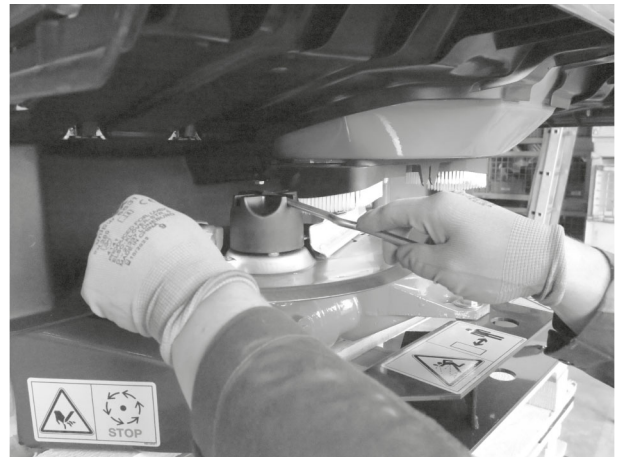
Afb. 78: Dopmoer losmaken
