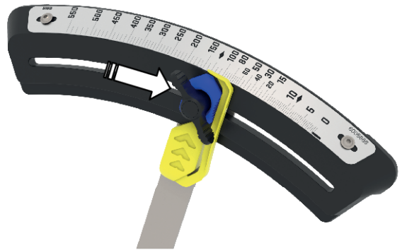
Afb. 75: Aanslag verschuiven
