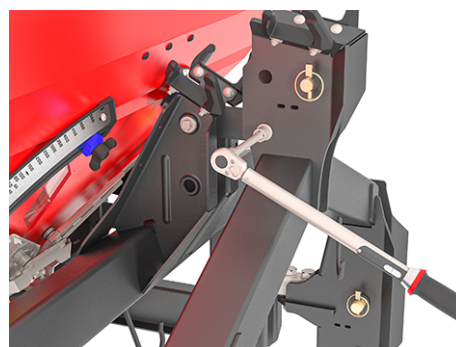
Afb. 66: Bevestiging van de trekstaaf aan het weegframe
