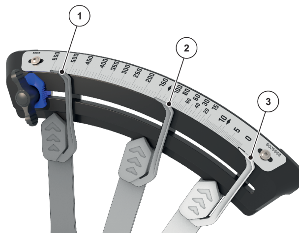
Afb. 31: Positioneren van de doseerschuif
