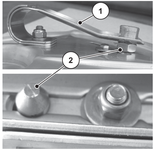
Afb. 79: Vergrendelingsbout naar behoren vergrendeld
