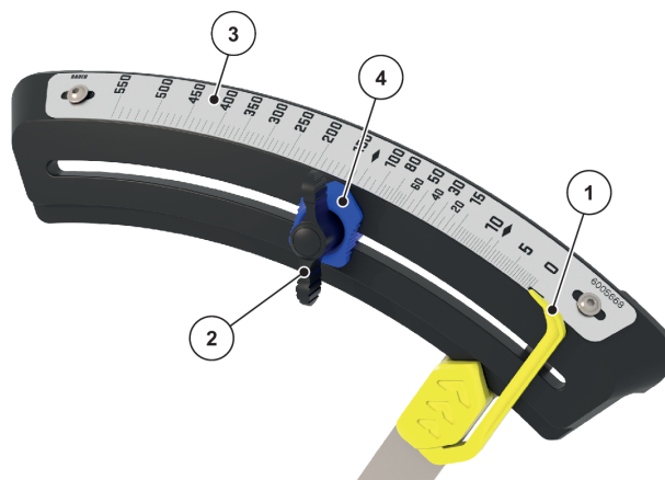
Afb. 41: Schaal voor instelling van de strooihoeveelheid (rijrichting rechts, varianten K/D/C)
