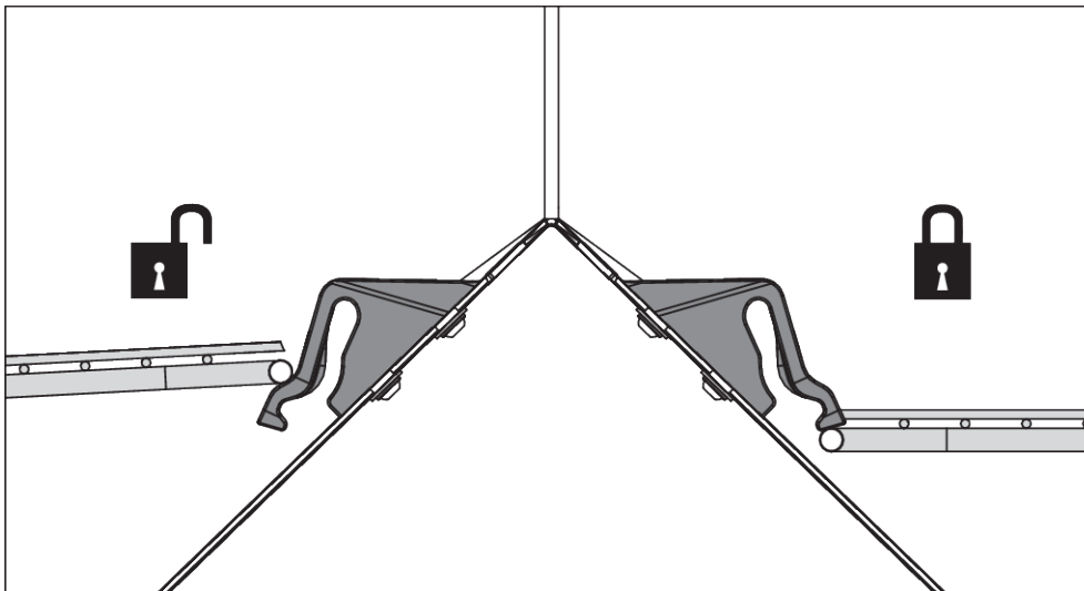
Afb. 67: Beschermroostervergrendeling open/gesloten
