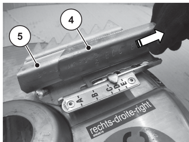
Afb. 84: Verlengings- en hoofdschoep
