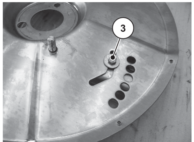
Afb. 90: Schroef aan de onderkant van de strooischijf
