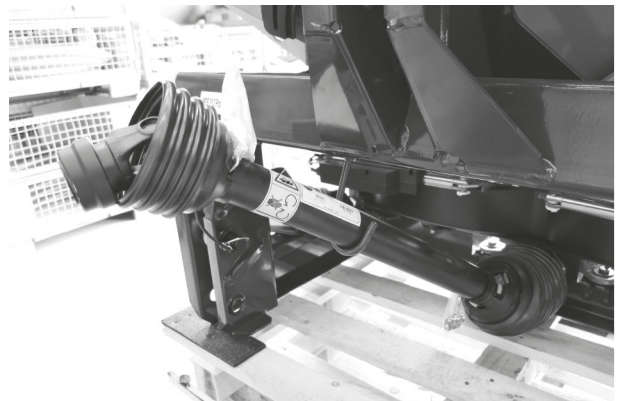
Afb. 18: Houder aftakas
