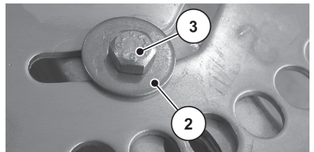
Afb. 94: Bevestigingspunten van de strooischoepen
