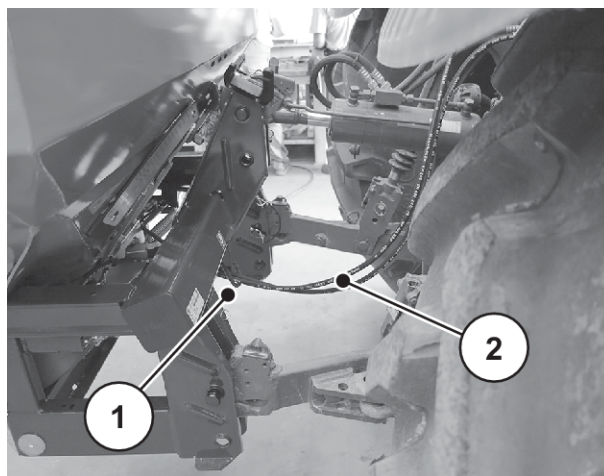
Afb. 25: Geleiding hydraulische slangen
