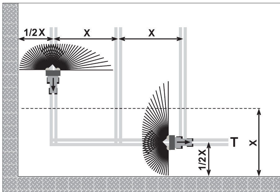
Afb. 59: Grensstrooien
