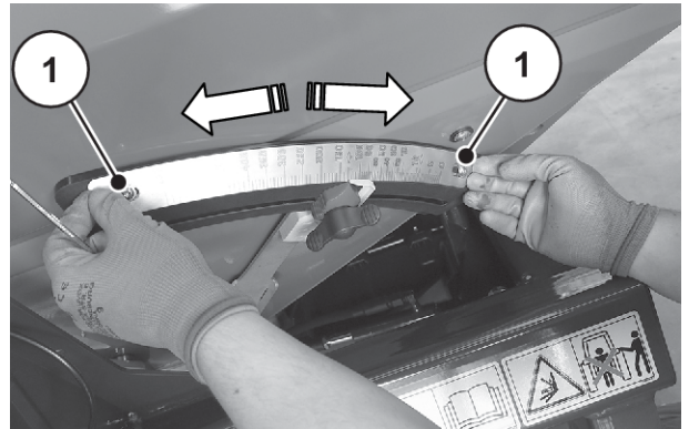
Afb. 76: Schaal verschuiven
