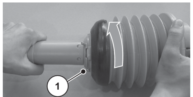
Afb. 19: Aftakasbescherming losmaken
