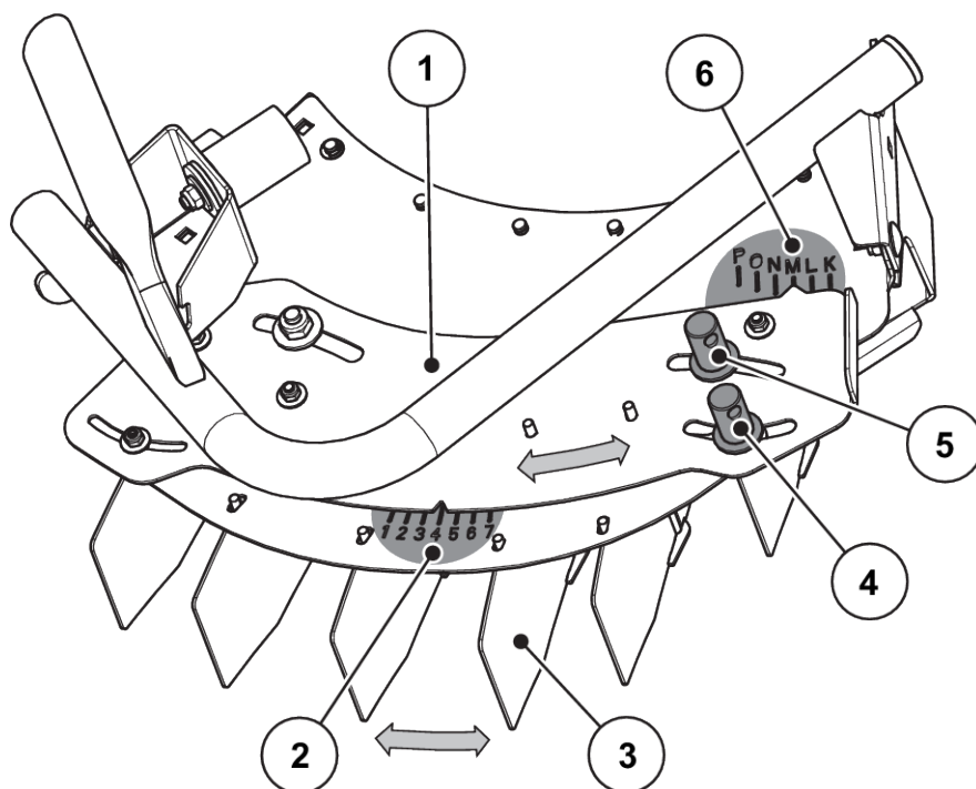
Afb. 57: TELIMAT Inrichting instellen
