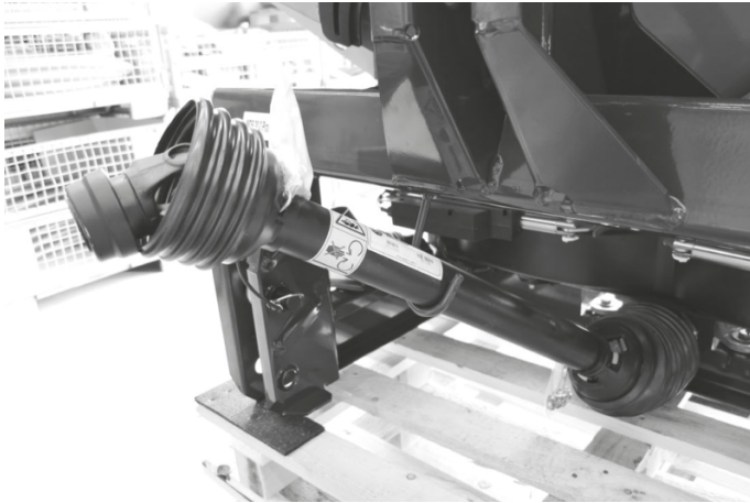
Afb. 64: Neerleggen van de aftakas, neerleggen van de kabels en hydraulische slangen
