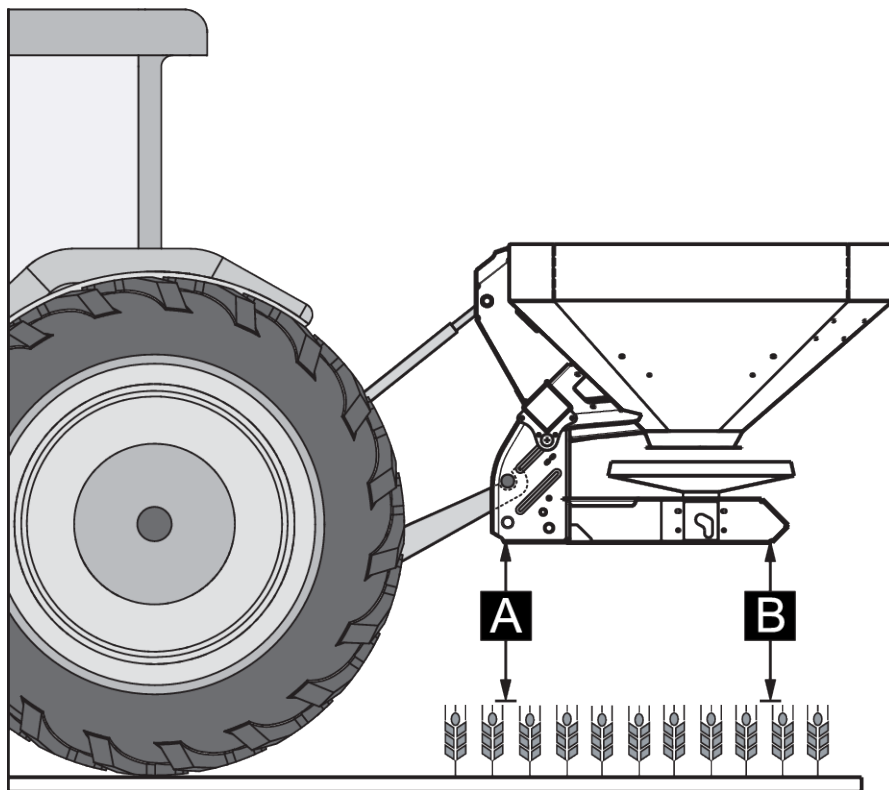
Afb. 27: Aanbouwpositie en -hoogte in de normale bemesting
