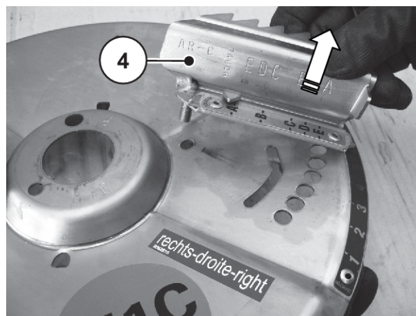
Afb. 91: Strooischoep verwijderen
