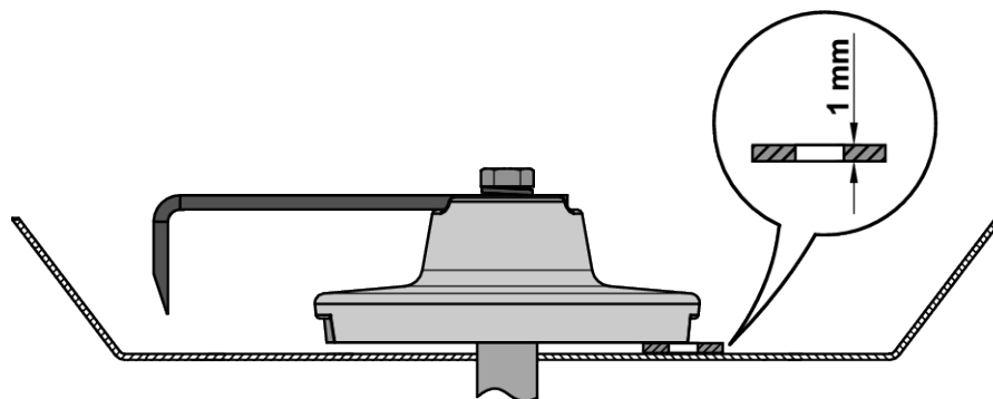
Afb. 80: Instelling van het roerwerk
