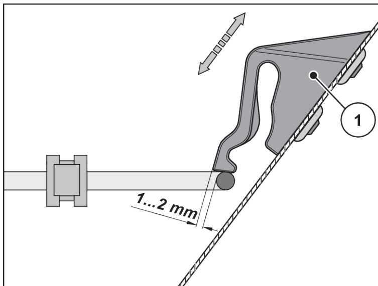
Afb. 69: Testmaat voor de functiecontrole van de vergrendeling van het beschermrooster
