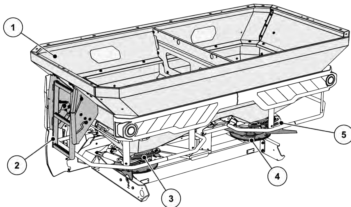
Fig. 6: Komponentoversikt: Bakside
