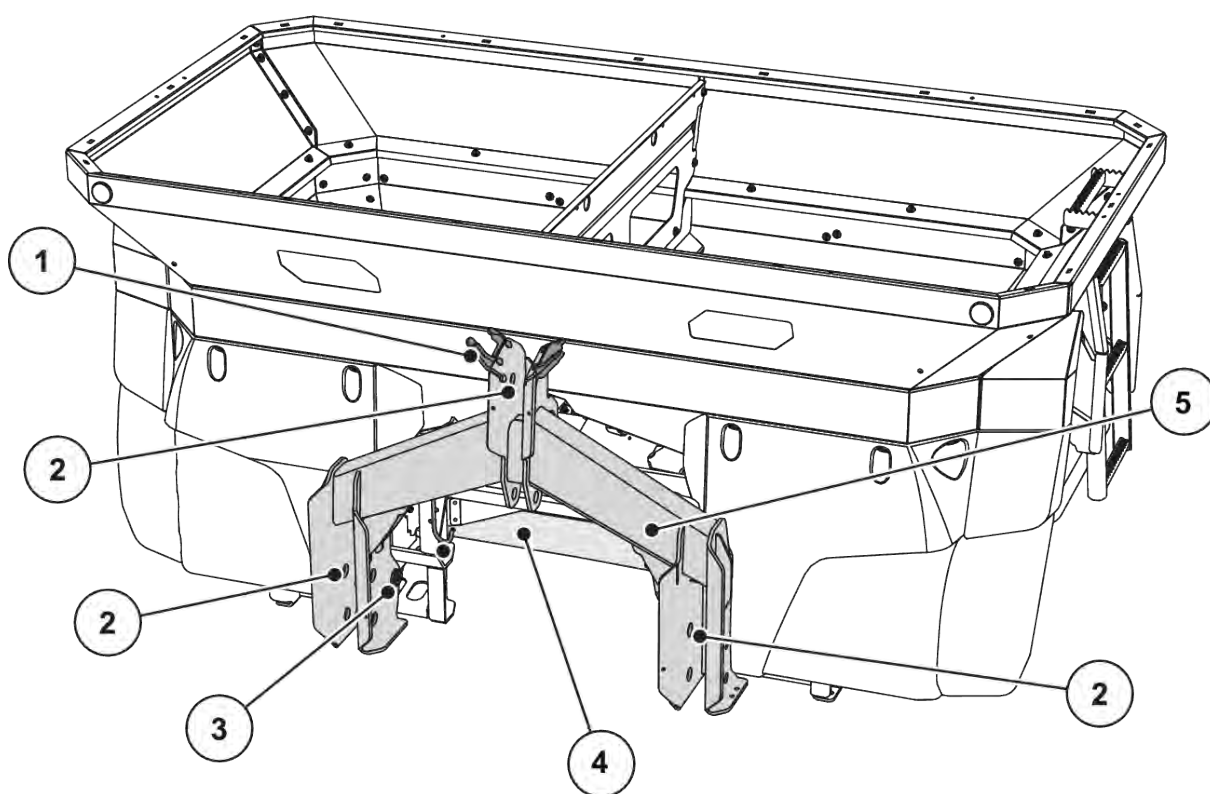
Fig. 5: Komponentoversikt: Forside
