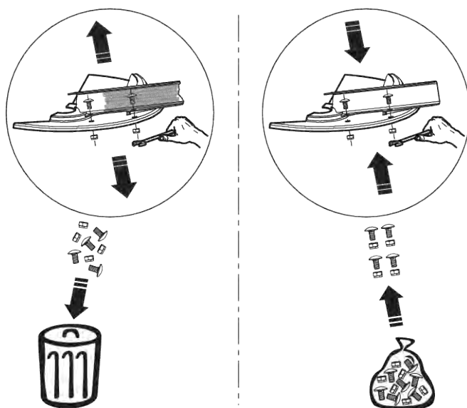
Fig. 57: Använd nya självlåsande muttrar.
