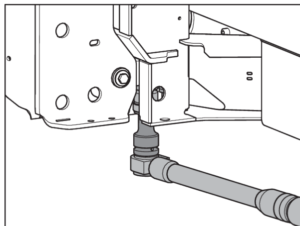
Fig. 45: Vägningscellens fastsättning (i färdriktning vänster)
