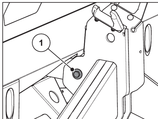
Fig. 46: Fastsättning av dragstången vid vägningsramen
