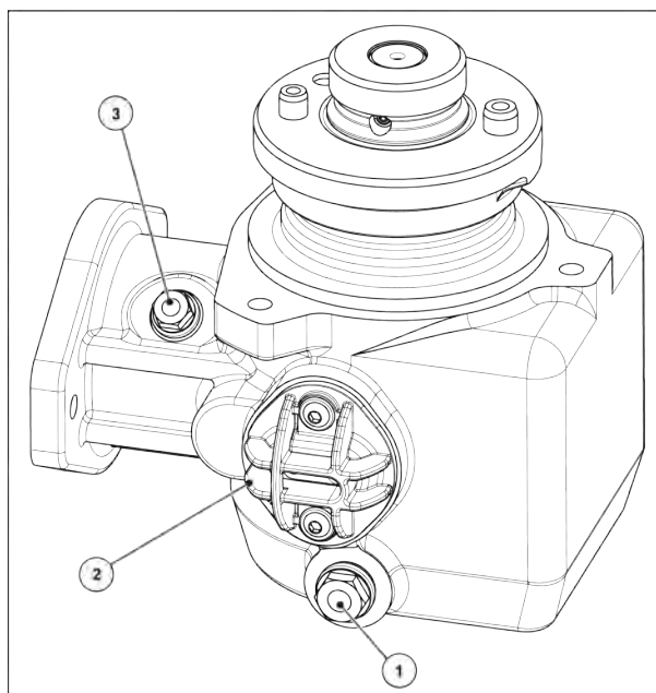
Att. 68: Transmisijas eļļas iepildīšanas un iztecināšanas vietas
