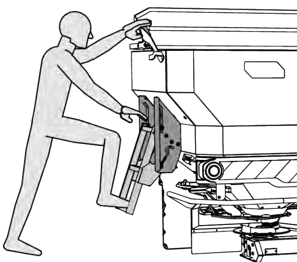
Ilust. 43: Escalera con lona de protección del depósito
