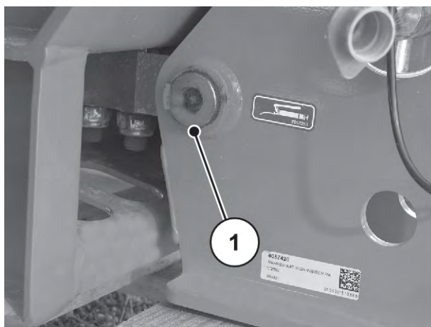
Ilust. 65: Punto de lubricación abonadora con sistema de pesaje
