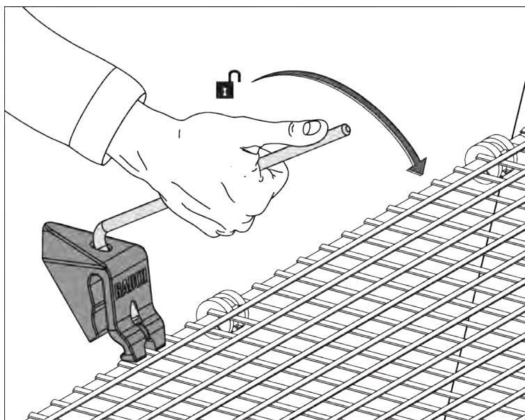
Ilust. 50: Abra el cierre de la rejilla de protección
