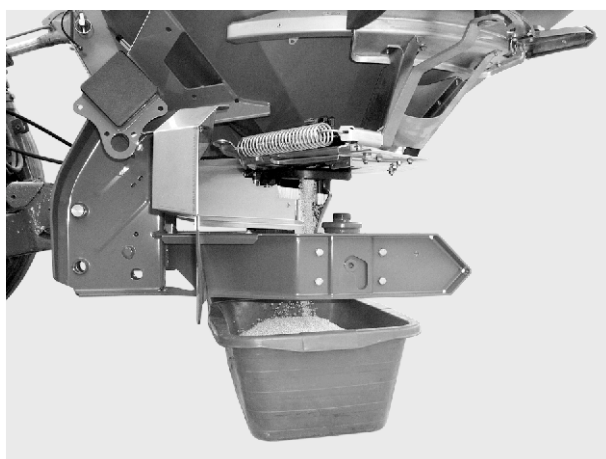
Fig. 39: Genomföra vridprov
