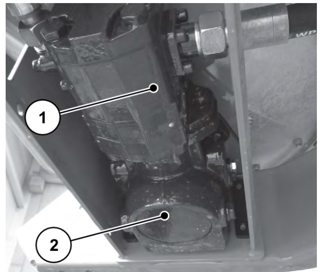
Fig. 66: Hydraulmotor
