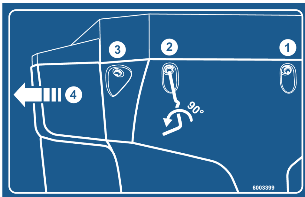
Fig. 52: Autocolant cu instrucțiuni colector de impurități
