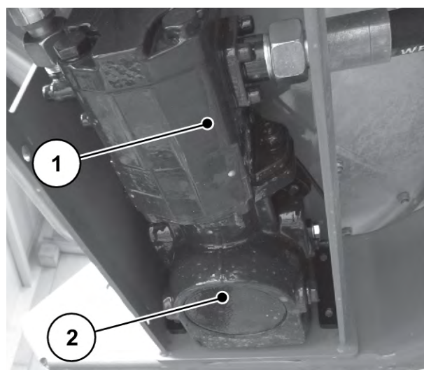
Fig. 66: Motor hidraulic
