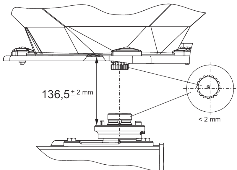
Fig. 53: Verificați poziția butucului discului aruncător
