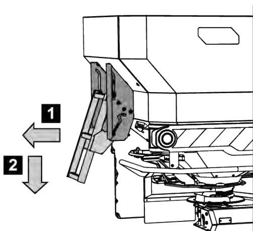
Rys. 44: Rozkładanie drabinki
