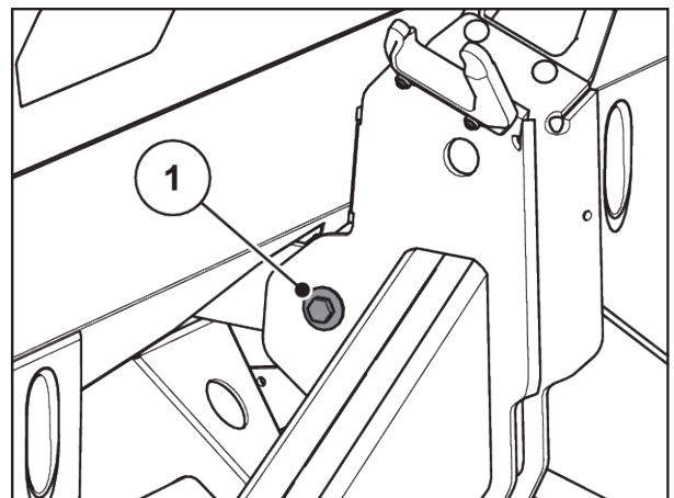
Rys. 47: Mocowanie ciągła do ramy wagi
