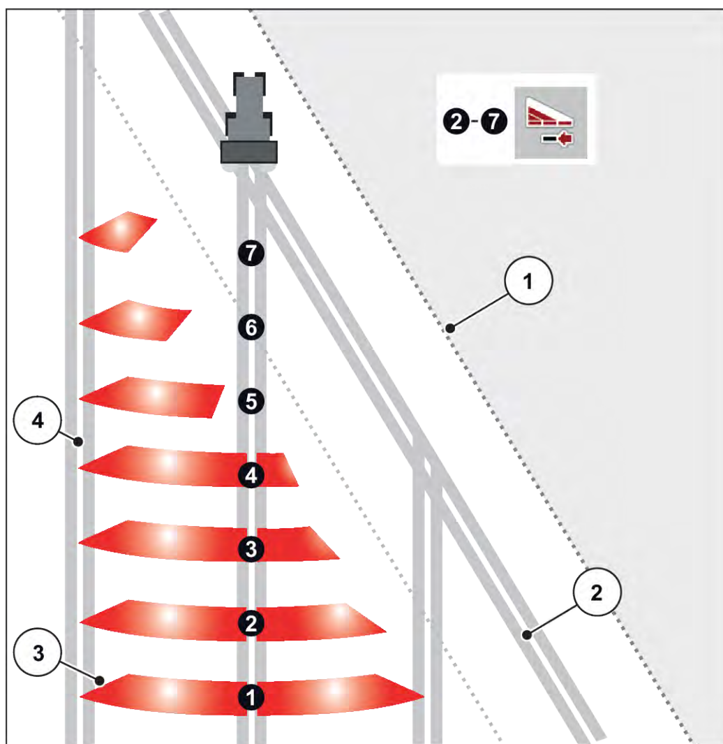
III. 33: Esempio di attivazione delle larghezze laterali con VariSpread pro
