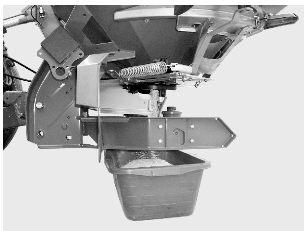
Ill. 39: Esecuzione del test di taratura
