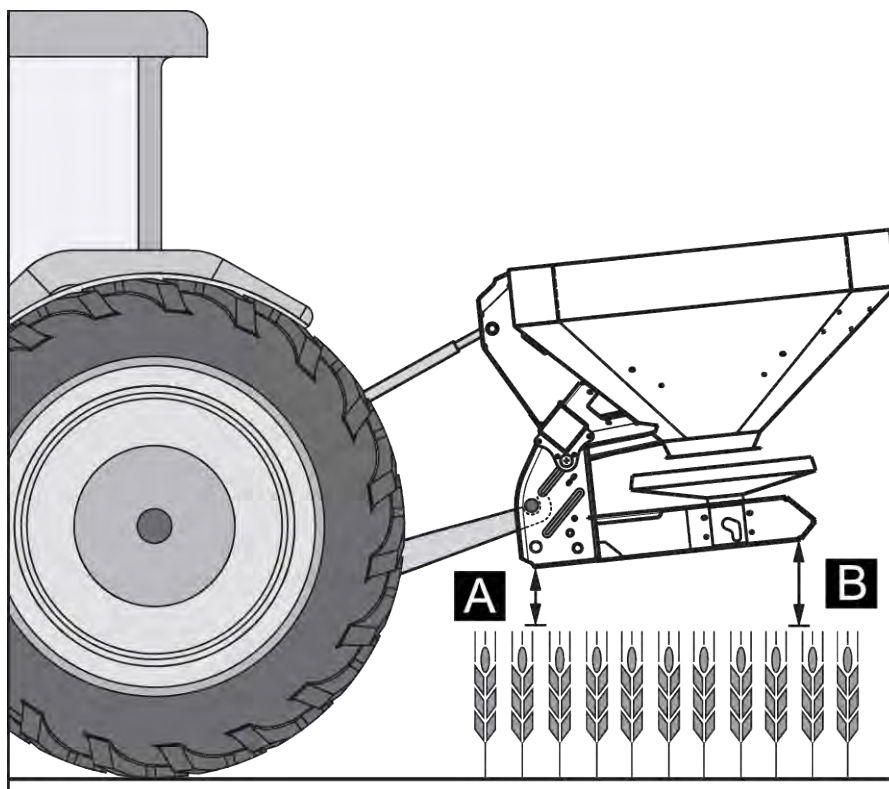
III. 17: Posizione e altezza di montaggio nella concimazione tardiva
