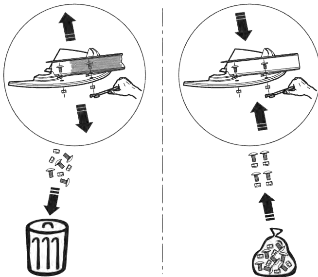
III. 58: Utilizzo di dadi autobloccanti nuovi
