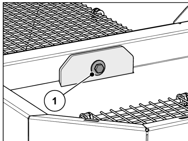
III. 48: Fissaggio della barra di trazione nel serbatoio
