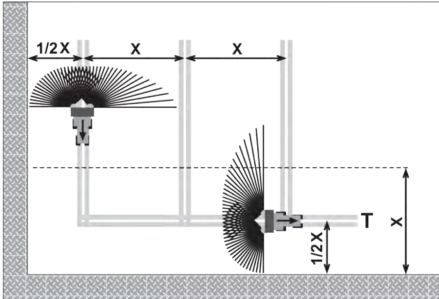
III. 31: Spargimento ai margini
